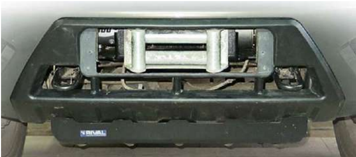
Кронштейн лебедки в штатный бампер (установка за номером) все кроме Diesel L.6302.1
